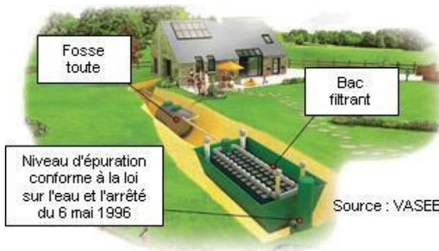
Représentation d'un système filtrant à zéolite
