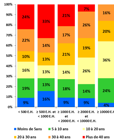
Âge des stations d'épuration
