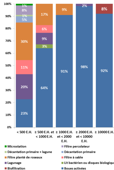
Répartition des procédés de traitement par taille de dispositif
