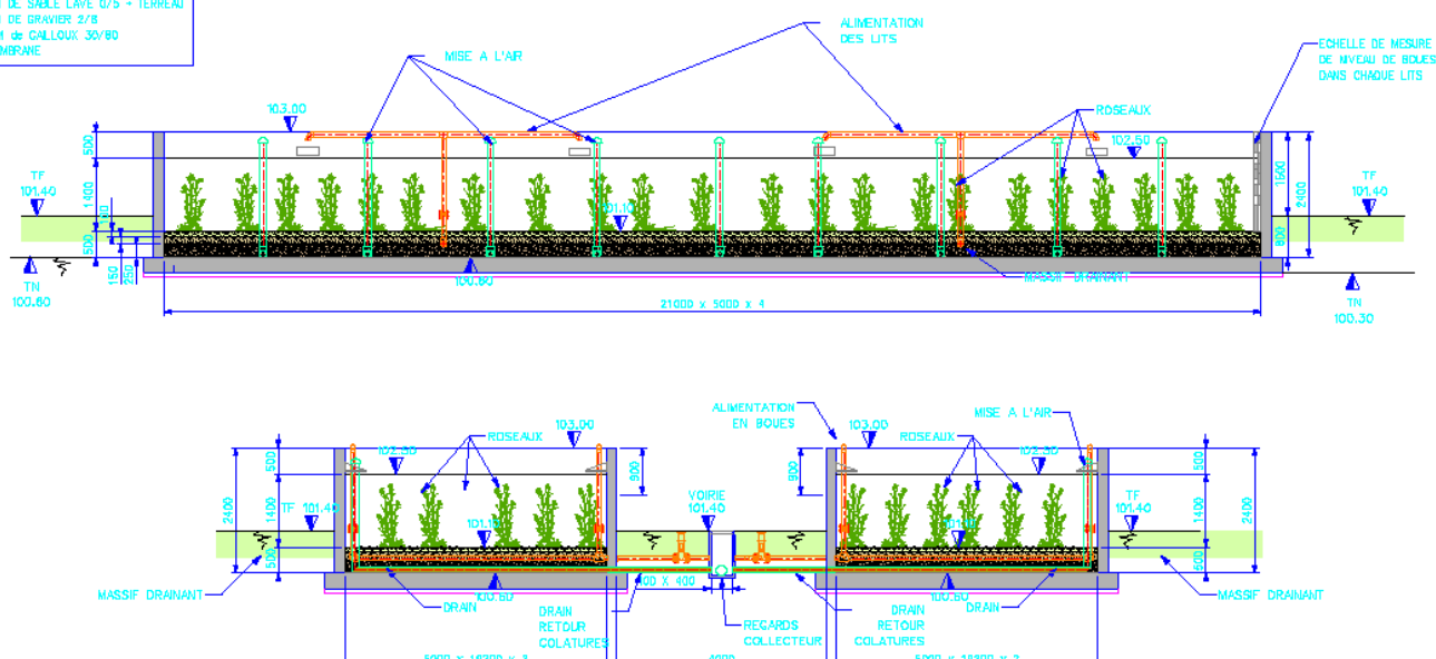
Rhizocompostage sur la commune de Touquin, avec ouvrages en béton (Hydrea)
