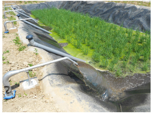
Lit planté de roseaux avec géomembrane
